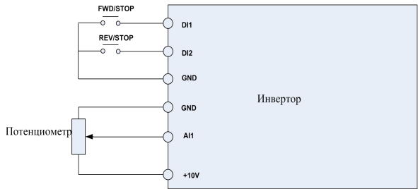
Рисунок 4 Монтаж выводов управления
