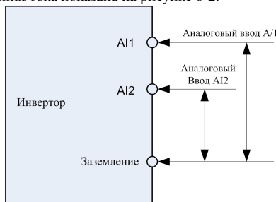
Рисунок 6-2 Схема для аналогового входа с внешним питанием
