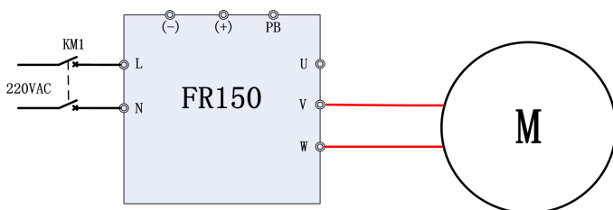
Рис. 6-20 Схема соединительного провода FR150 и однофазного двигателя (убрать конденсатор)
