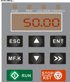
Рисунок 7 Внешний вид панели управления
