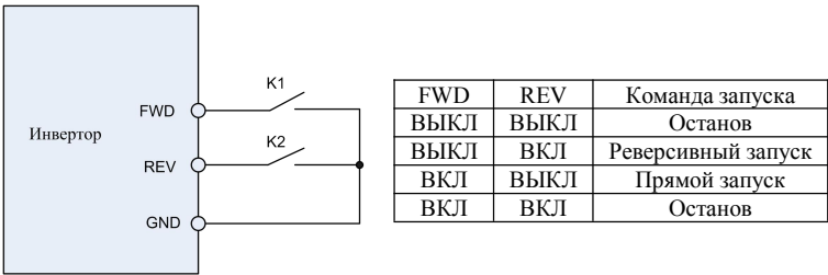
Рисунок 6-8 Установка двухпроводного режима 1
