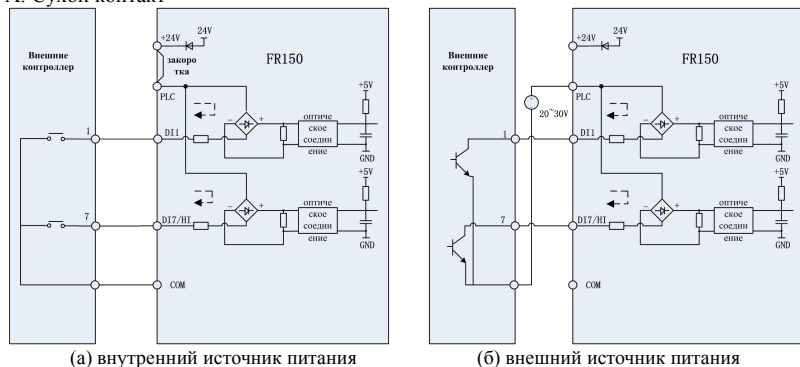
Рис. 3-11 Сухой контакт
