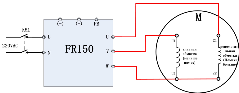
Рис. 6-18 Схема соединительного провода FR150 и однофазного двигателя прямого вращения (убрать конденсатор)
