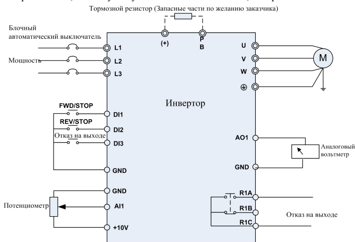
Рисунок 6 Объединенная схема
