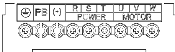
Рис. 3-8 Выводы цепи питания трехфазного инвертора FR150
