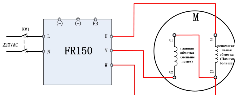
Рис. 6-19 Схема соединительного провода FR150 и однофазного двигателя (убрать конденсатор)
