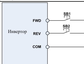
Рисунок 6-12 Схема управления импульсной операцией останова
