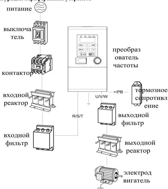
Рис.3-4 Стандартная конфигурация периферийных устройств
