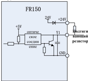
(а) внутренний источник питания
