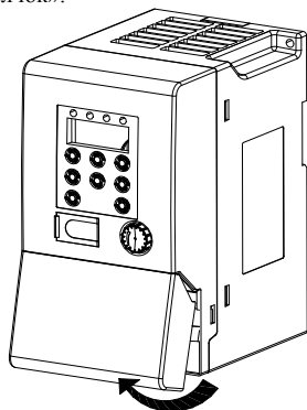
(а) Снятие крышки клемм
