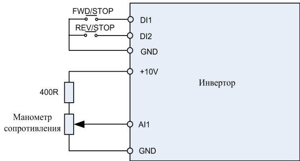
Рисунок 5 Монтаж выводов управления
