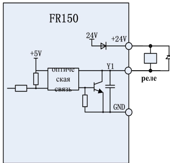
(а) внутренний источник питания
