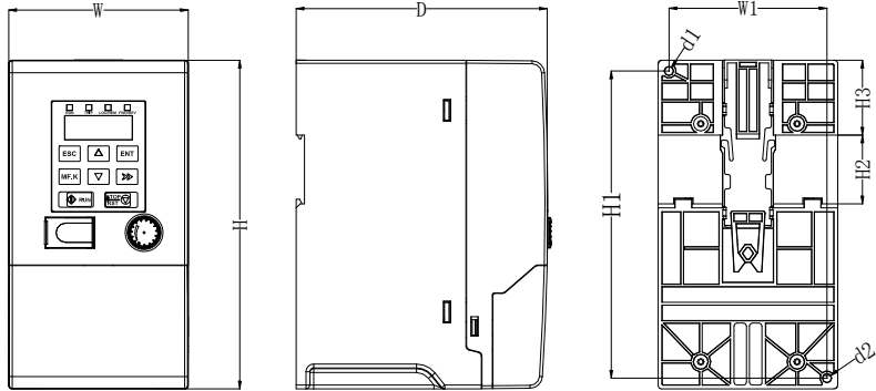
Fig 2-4 Габариты клавиатуры
