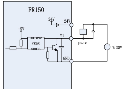
(б) внешний источник питания
