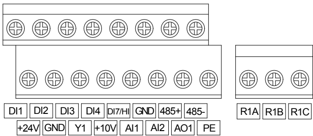
Рисунок 3 Схемы выводов управления серии FR150
