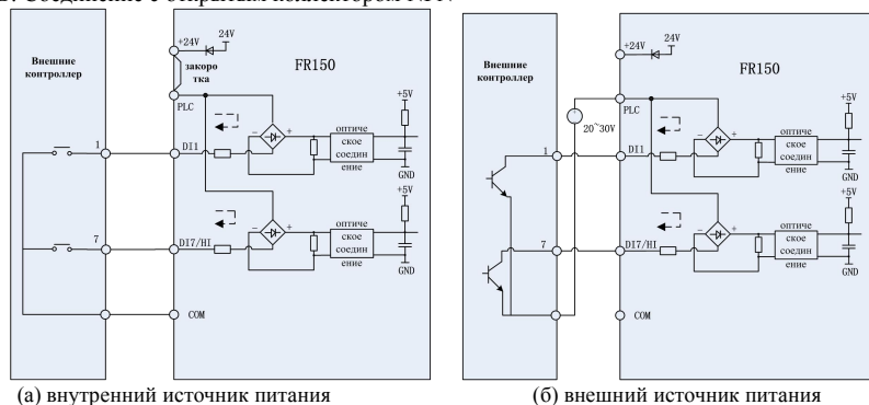
Рис. 3-12 Соединение с открытым коллектором NPN
