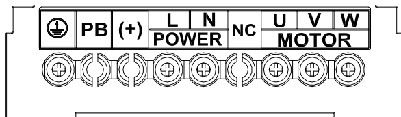
Рис. 3-7 Выводы цепи питания однофазного FR150
