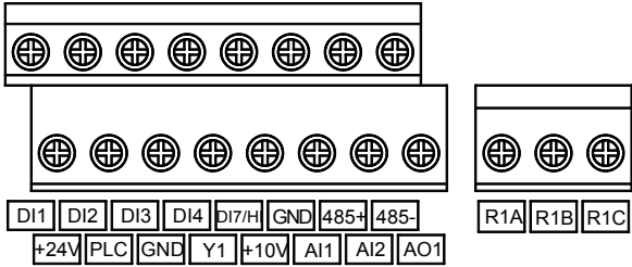
Рис. 3-9 Клеммы цепи управления
