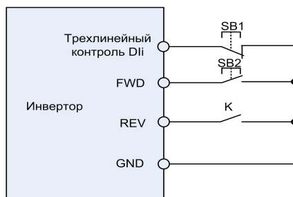
Рисунок 6-11 Настройка трехпроводного управления 2
