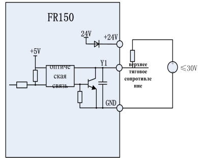
(б) внешний источник питания
