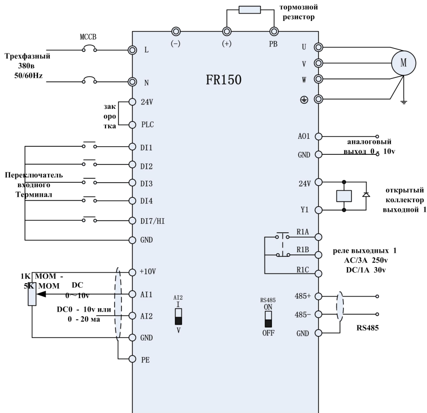
Рис. 3-6 Монтажная схема трехфазного преобразователя 380 В
