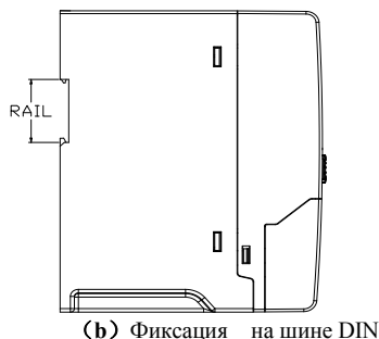
Рис. 3-1 Методы установки
